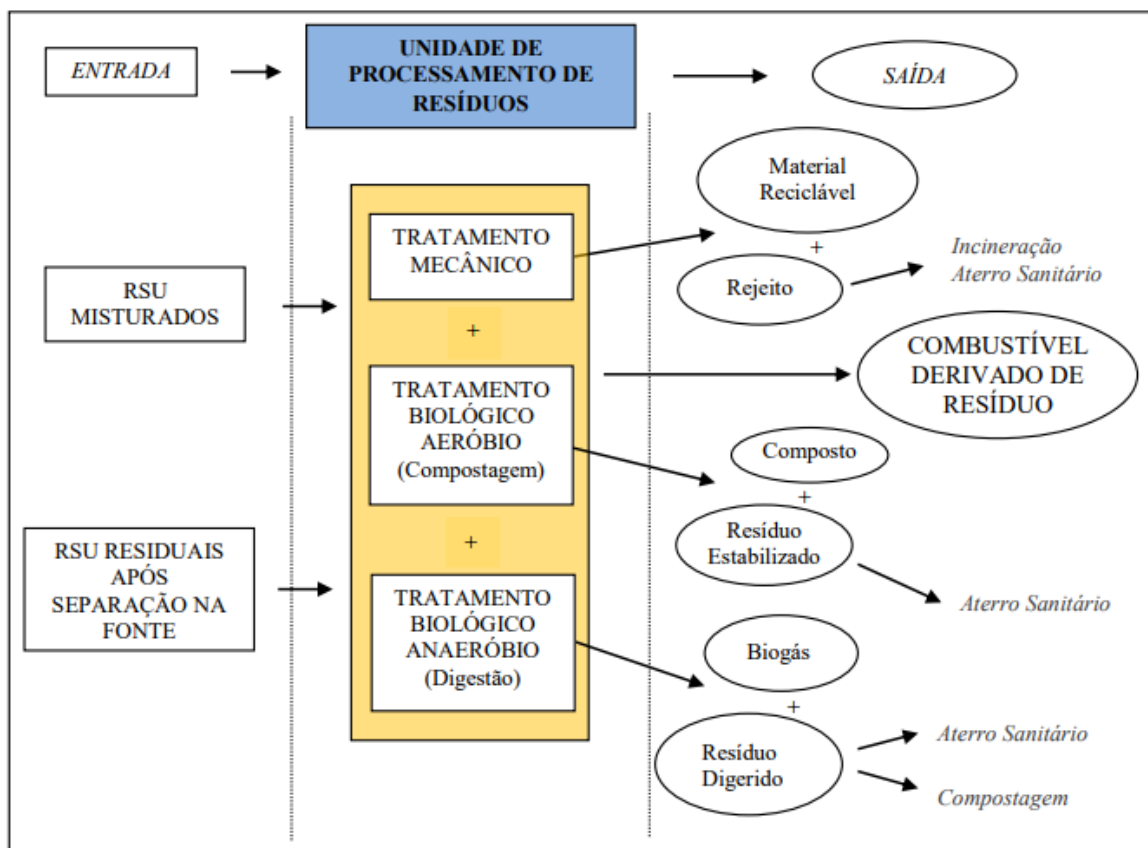
Figura 4: Diferentes fluxos de entradas e saídas adotados em uma UPR
