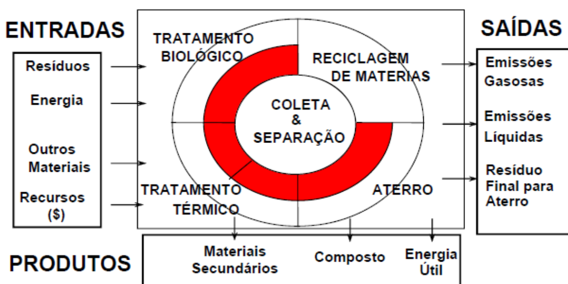
Figura 8: Limites do sistema para o Inventário do Ciclo de Vida
