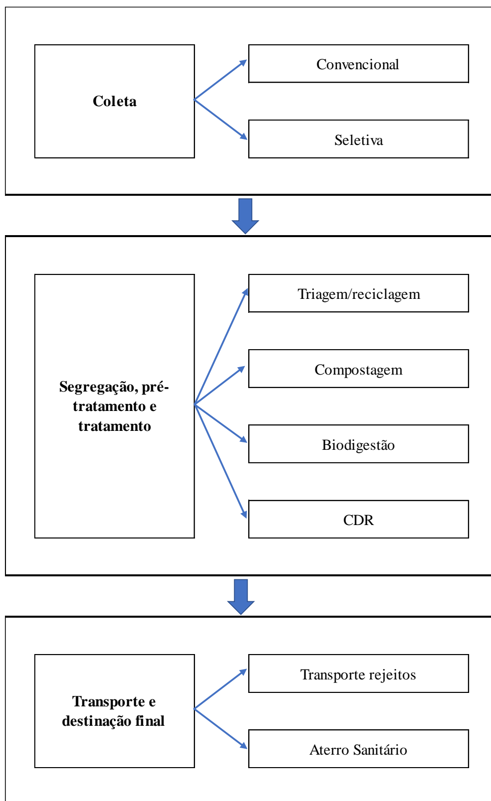
Figura 19: Etapas de gerenciamento de RSU que poderão compor as rotas tecnológicas para os cenários.
