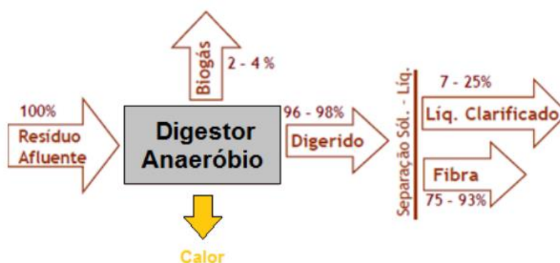
Figura 3: Balanço de massa típico de um sistema de DA (percentagens mássicas)
